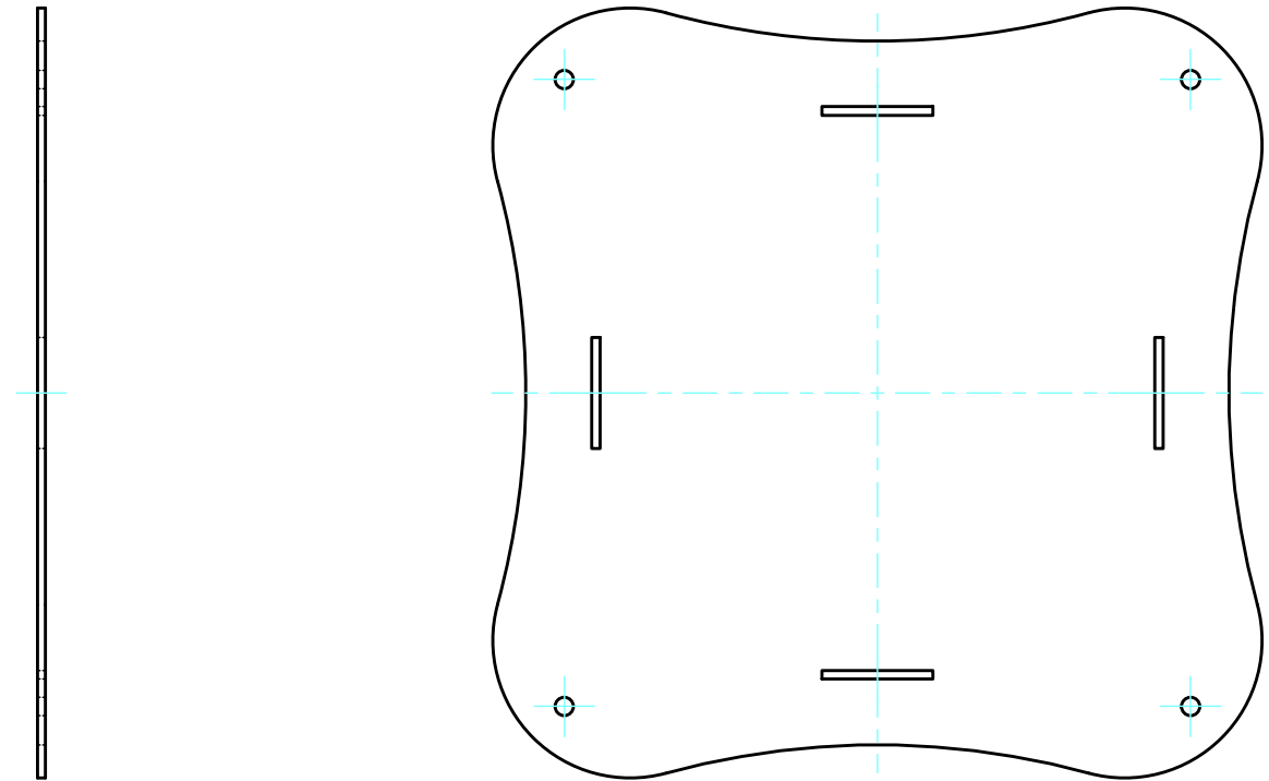
下カバー裏面 / Bottom cover Backside
