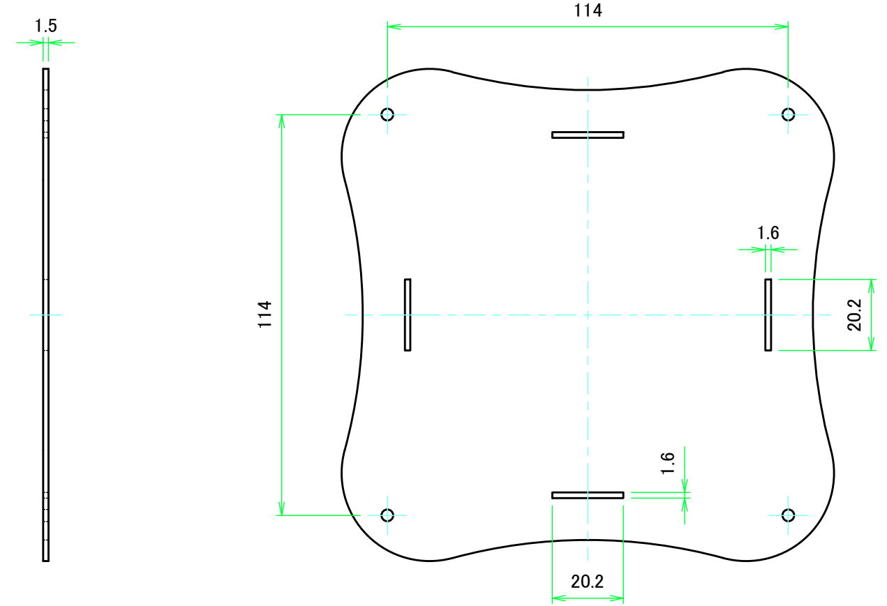
上カバー裏面 / Top cover Backside
